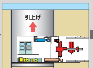
中胴押し出し・引き上げ
