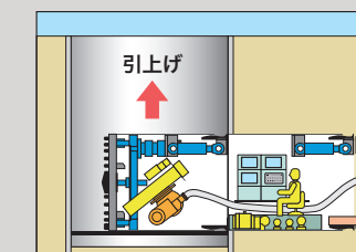
前胴押し出し・引き上げ
