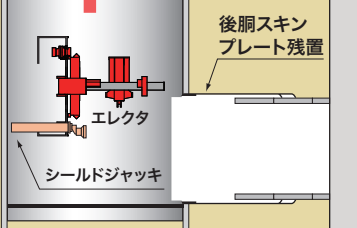
テール内部ユニット引き上げ・後胴スキムプレート残置
