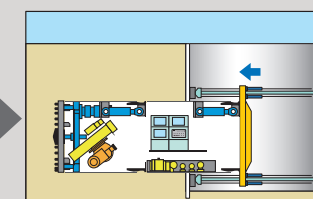
中胴接続・掘進
