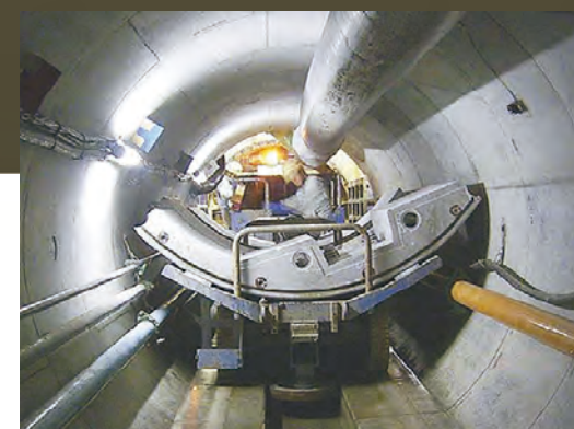
セグメント坑内搬送システム
