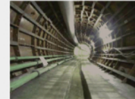
曲線部施工状況
